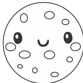
Mercurio
