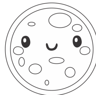
Neptuno
