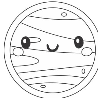
Júpiter
