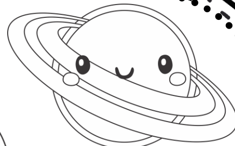
Saturno
