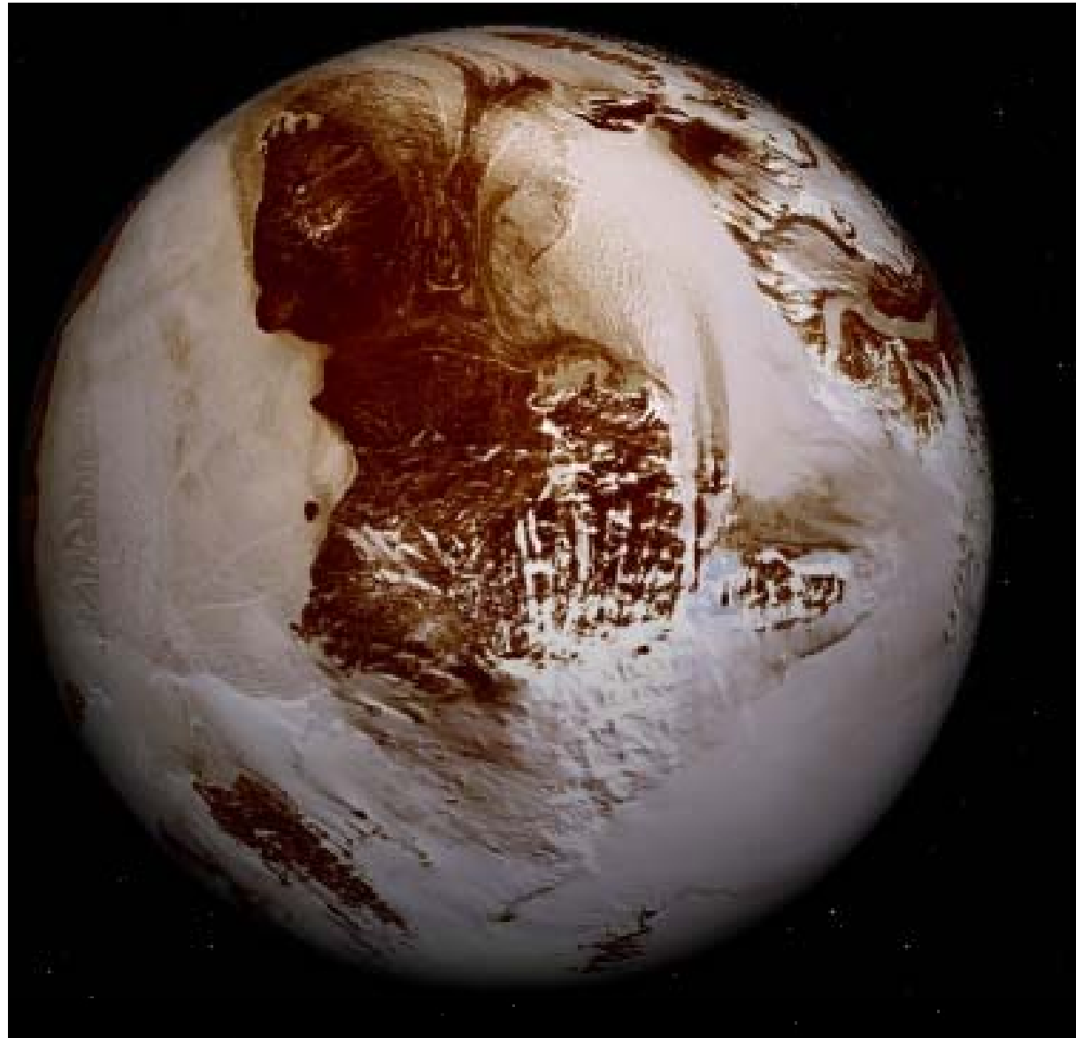
Plutón
