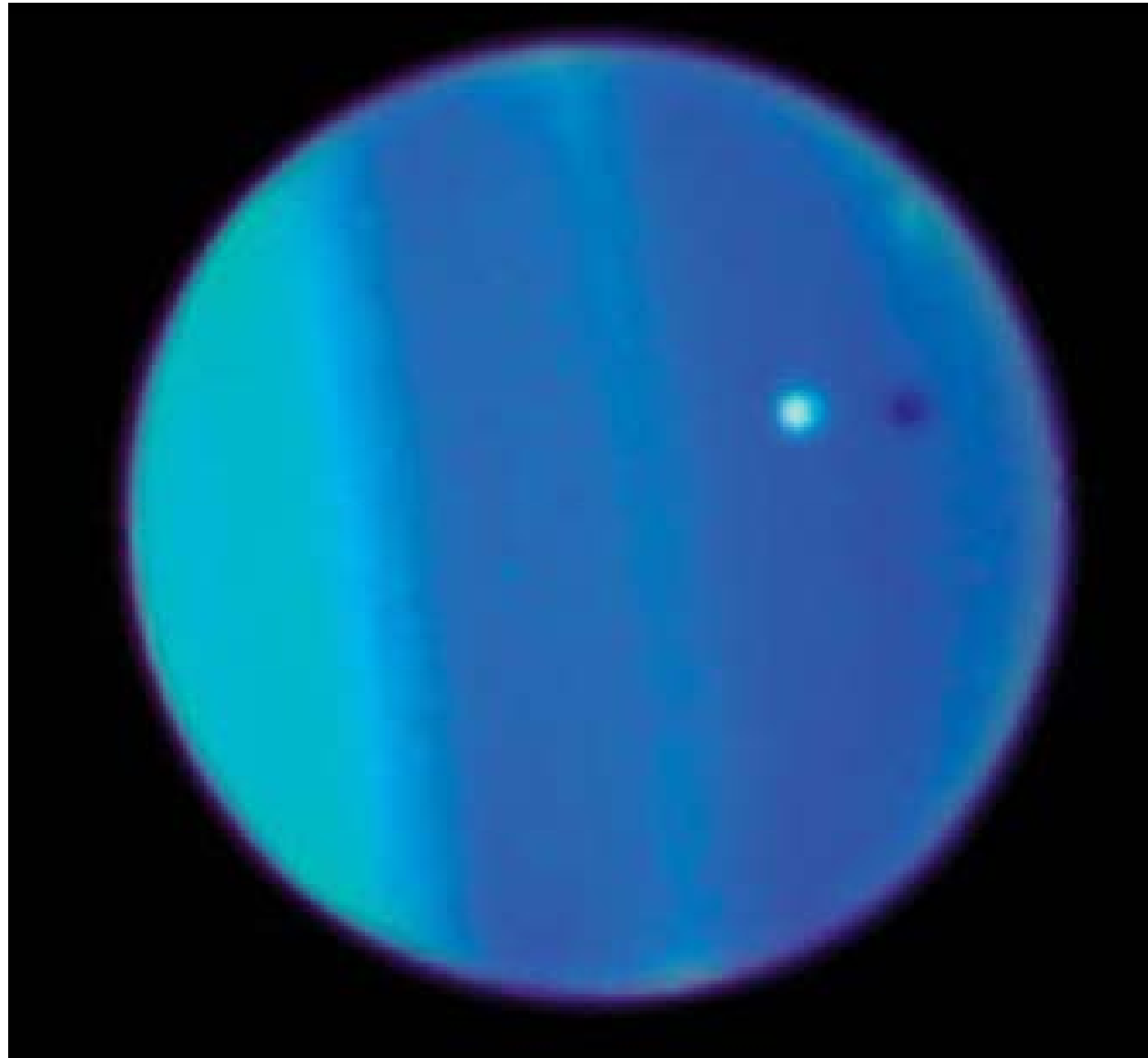
Urano
