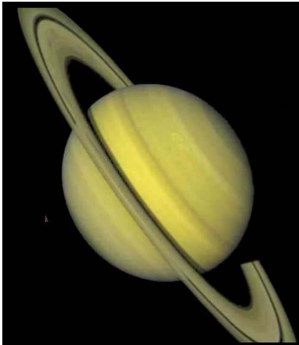
Saturno
