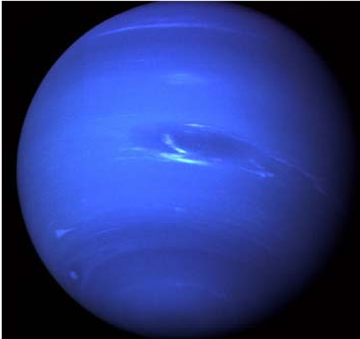
Neptuno
