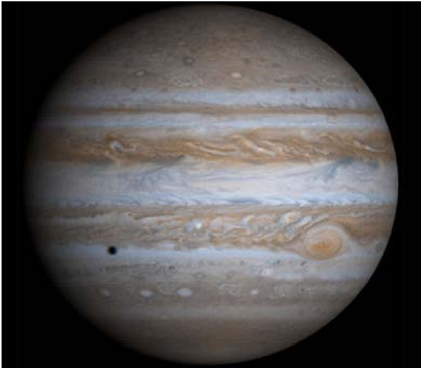
Júpiter
