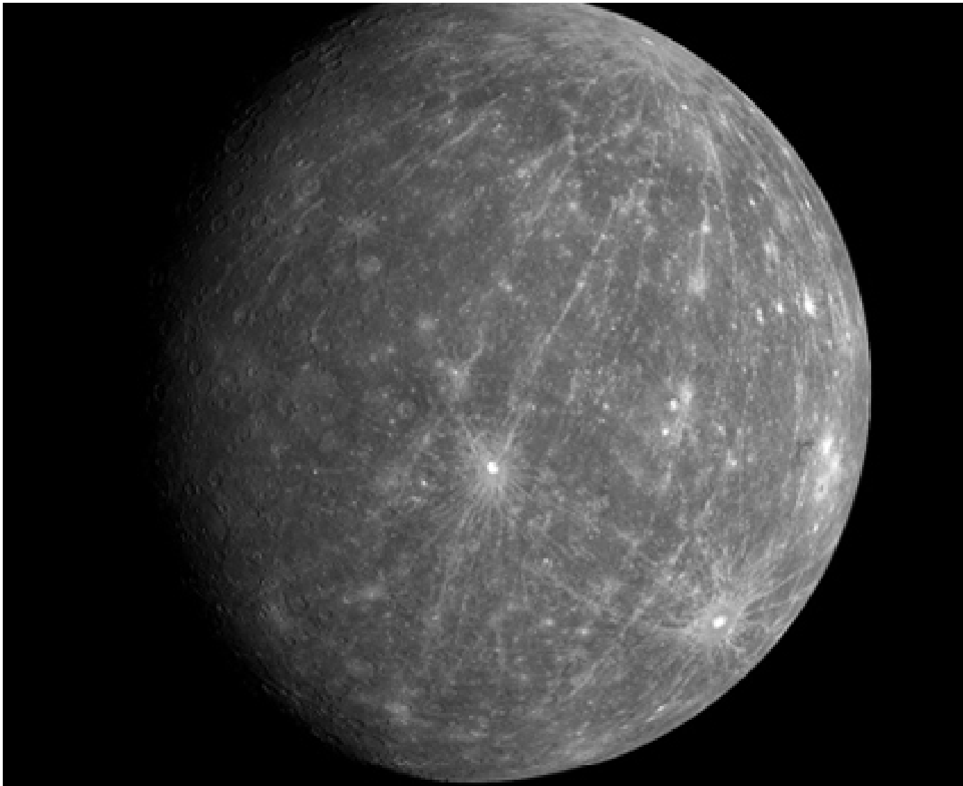
Mercurio
