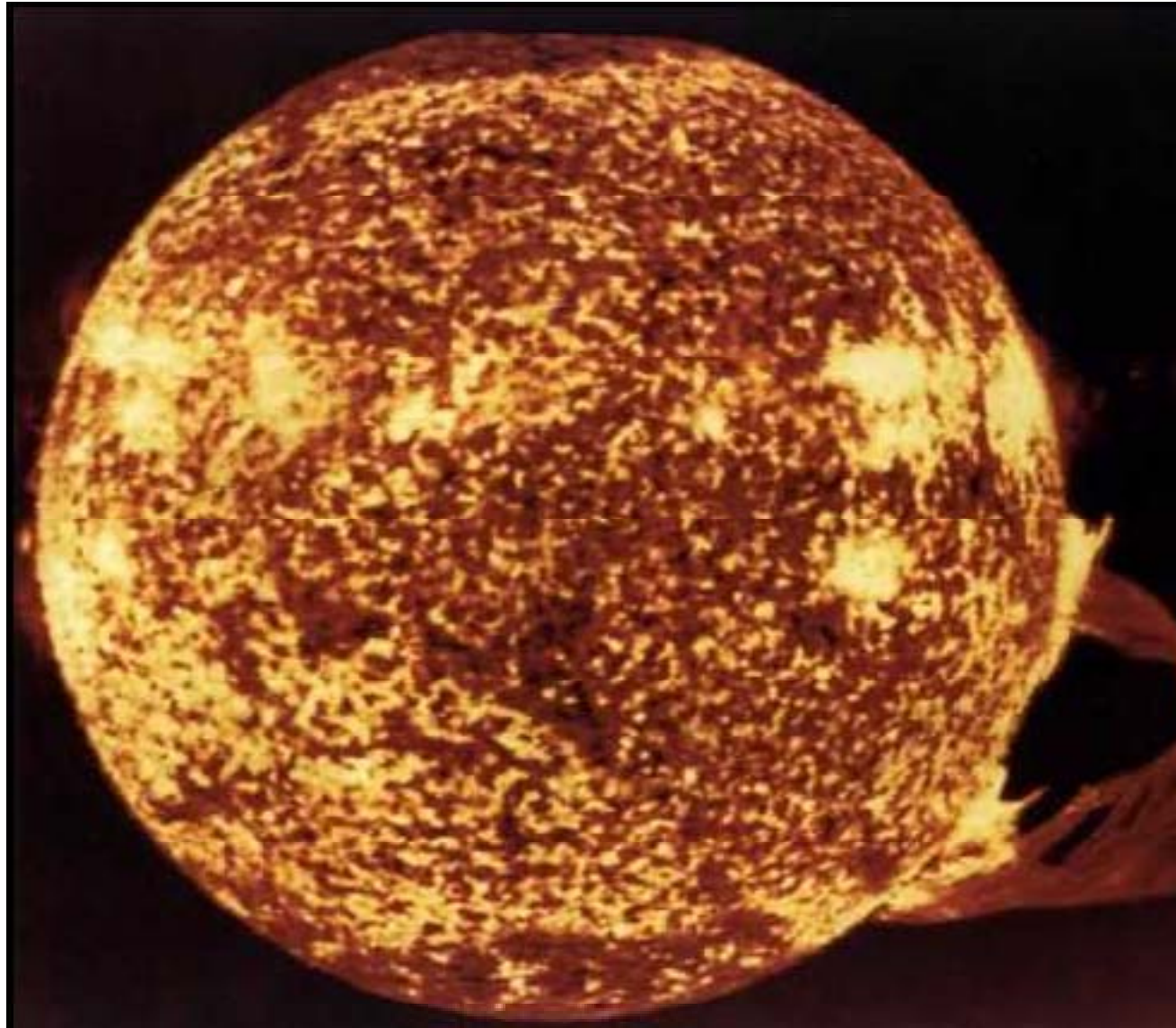
El sol
