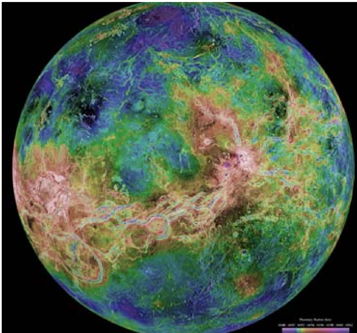
Venus
